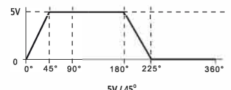
Çıkış sinyali
