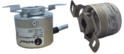
B-A-YH 50 Gövde Yarım Hellow Shaft (Yarım Delik)
